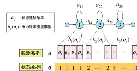
図 3 隠れマルコフモデル: HMM
