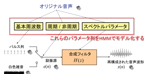
図 2 音声の分析と再構成
